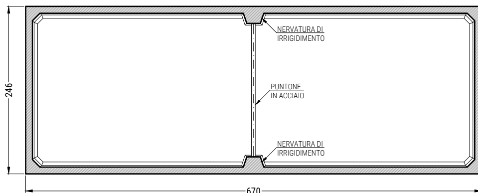
PIANTA COPERTURA
