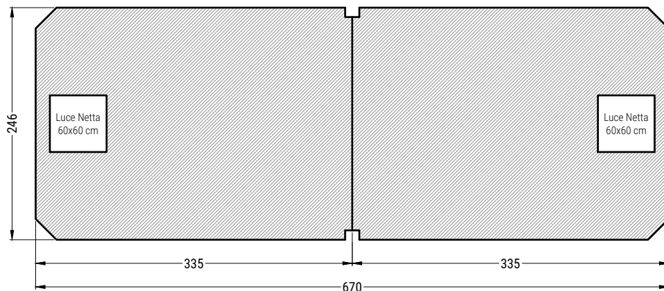
PIANTA COPERTURA
